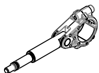
P2.150.002 PREMONTATO BIELLA - ASTA PER POMPA "PM"
